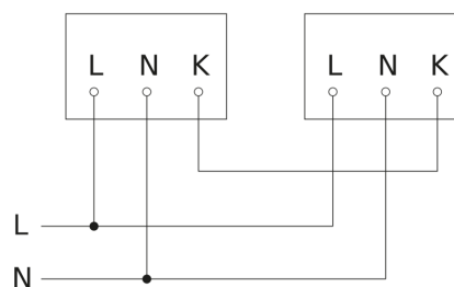
Diagrama electrónico interconexión maestro-maestro
